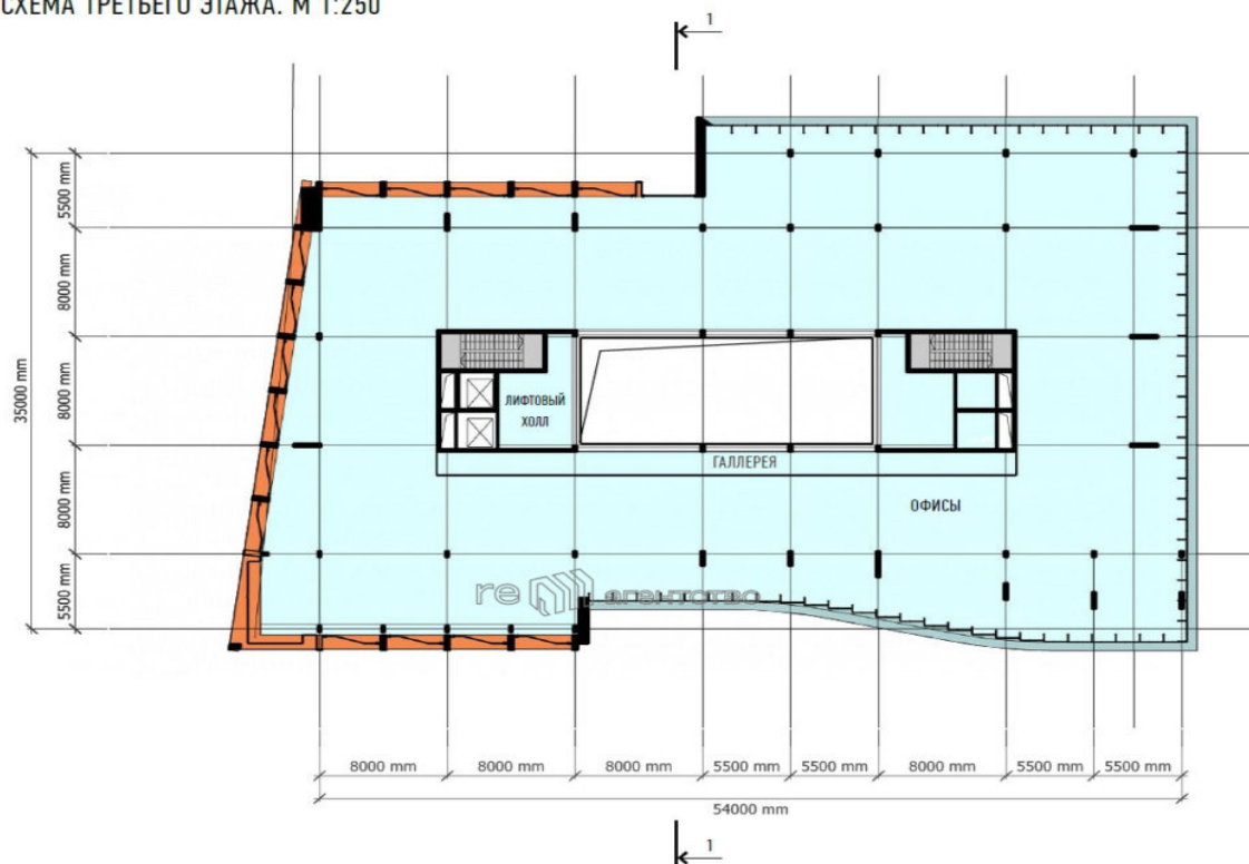
ПЛАН-СХЕМА ТРЕТЬЕГО ЭТАЖА. М 1:250
