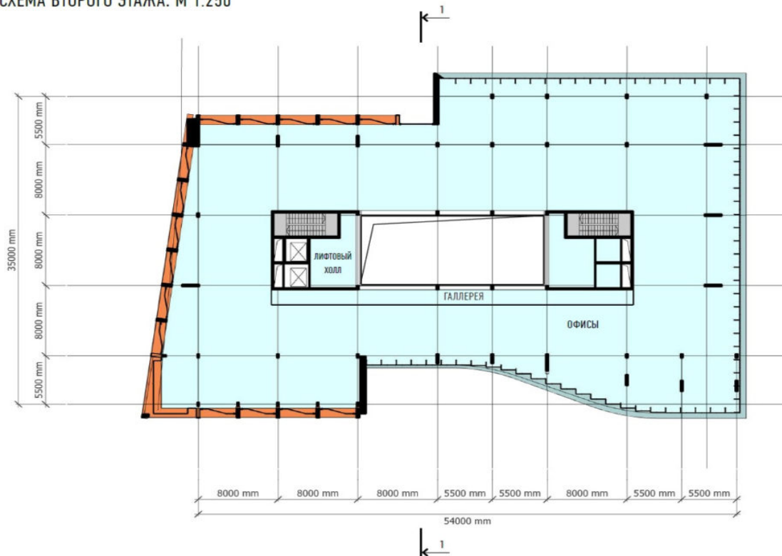
ПЛАН-СХЕМА ВТОРОГО ЭТАЖА. М 1:250
