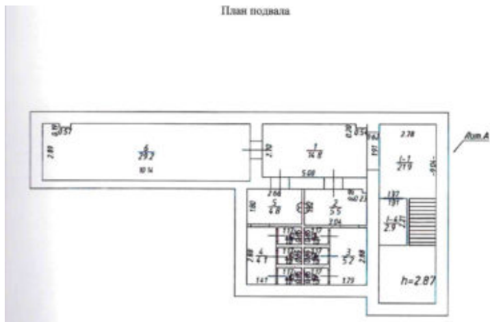
План подвала
